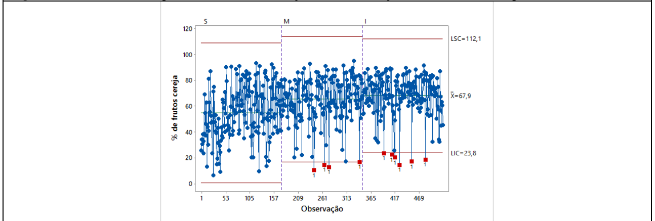
Figura 2. Carta de controle para o estágio de maturação cereja nos terços inferior, médio e superior.
